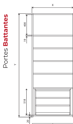
TYPE A [858 ; 958]
