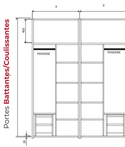
TYPE F [2064 ; 2464]
