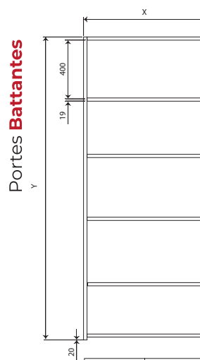
TYPE C [858 ; 1258]
