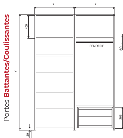
TYPE E [1470 ; 2464]
