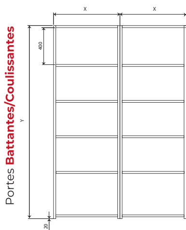
TYPE D [1470 ; 2464]
