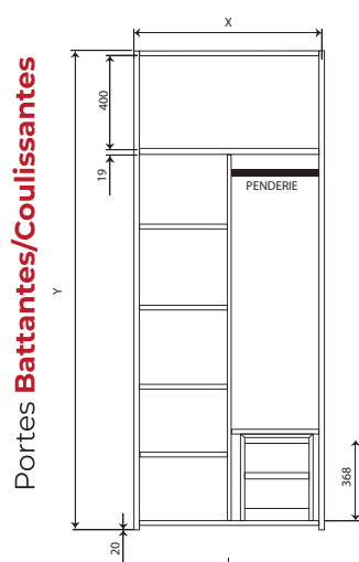
TYPE B [1058 ; 1258]
